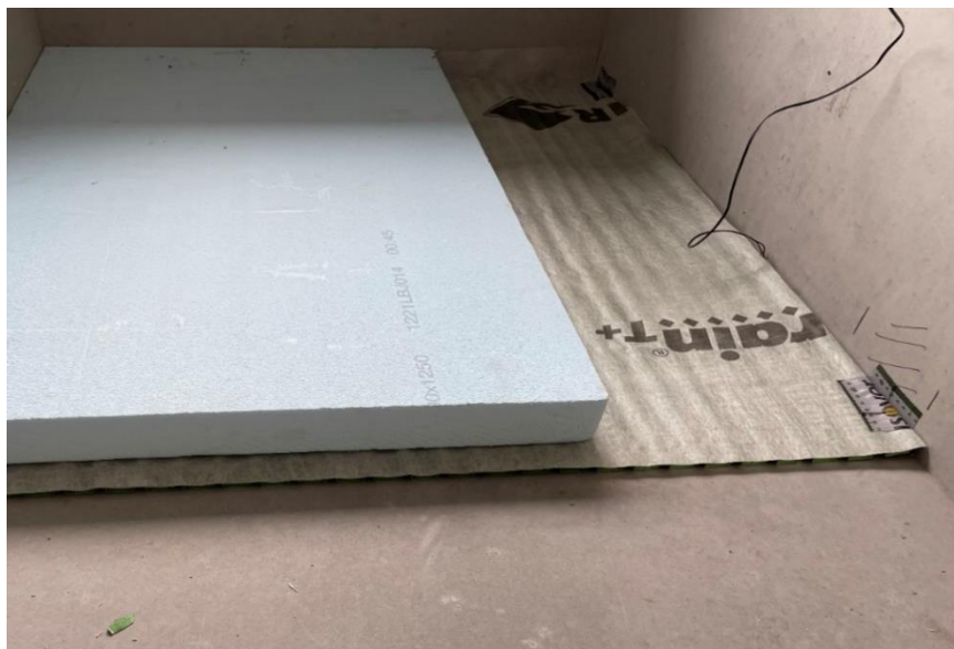
Abb. 5: Beispiel einer Drainagematte (AquaDrain T+) sowie Wärmedämmung aus XPS vor Einbau des Zementestrichs
